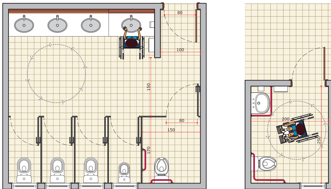
Na desenho da esquerda, exemplo de reforma de sanitário existente, e no desenho a direita, exemplo de novo banheiro. Fonte: acervo autoras
