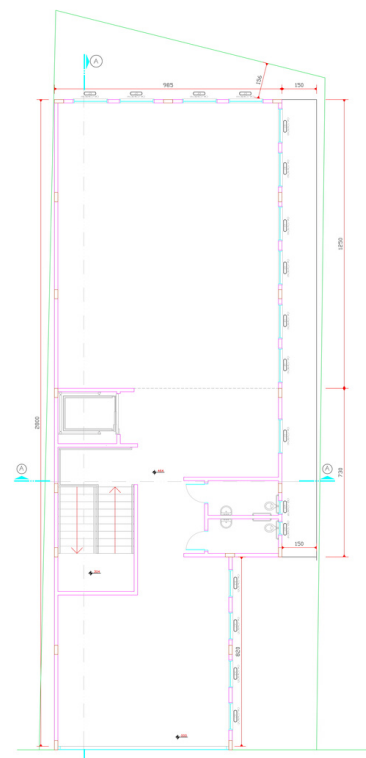
PLANTA BAIXA - 2º Piso Escala 1/50 Área Total: 258,17m 2
