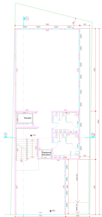
PLANTA BAIXA - 1º Piso Escala 1/50 Área Total: 258,17m 2
