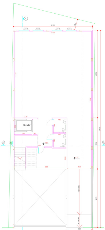
PLANTA BAIXA - Subsolo Escala 1/50 Área Total: 224,73m 2
